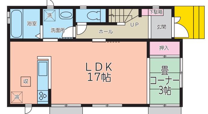
1階平面図:51.35㎡(15.53坪)
